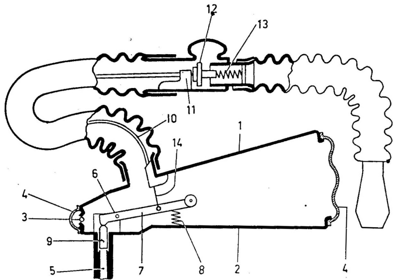
Schema di funzionamento dell'erogatore polmone dell'Explorer Standard.
