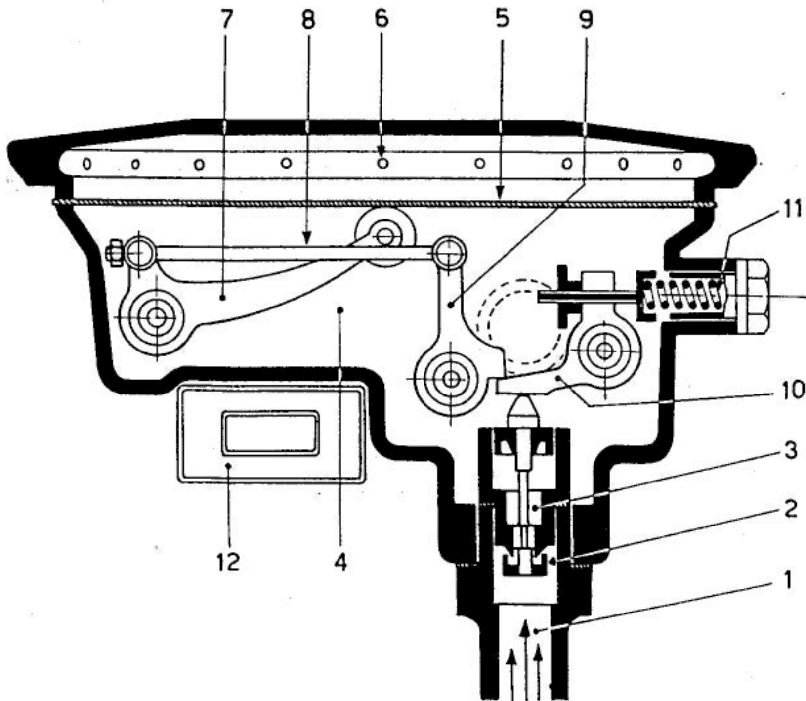
Schema di funzionamento dell'erogatore dell'Abissal Super.
